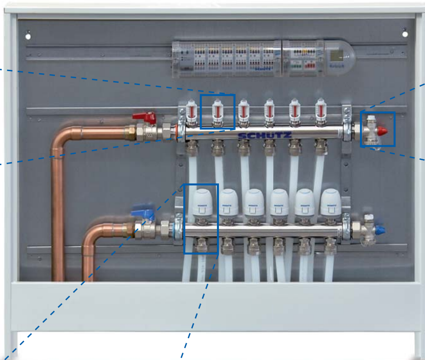
Vorlaufverteiler DN25 mit integrierter, drehbarer Durchflussanzeige.
